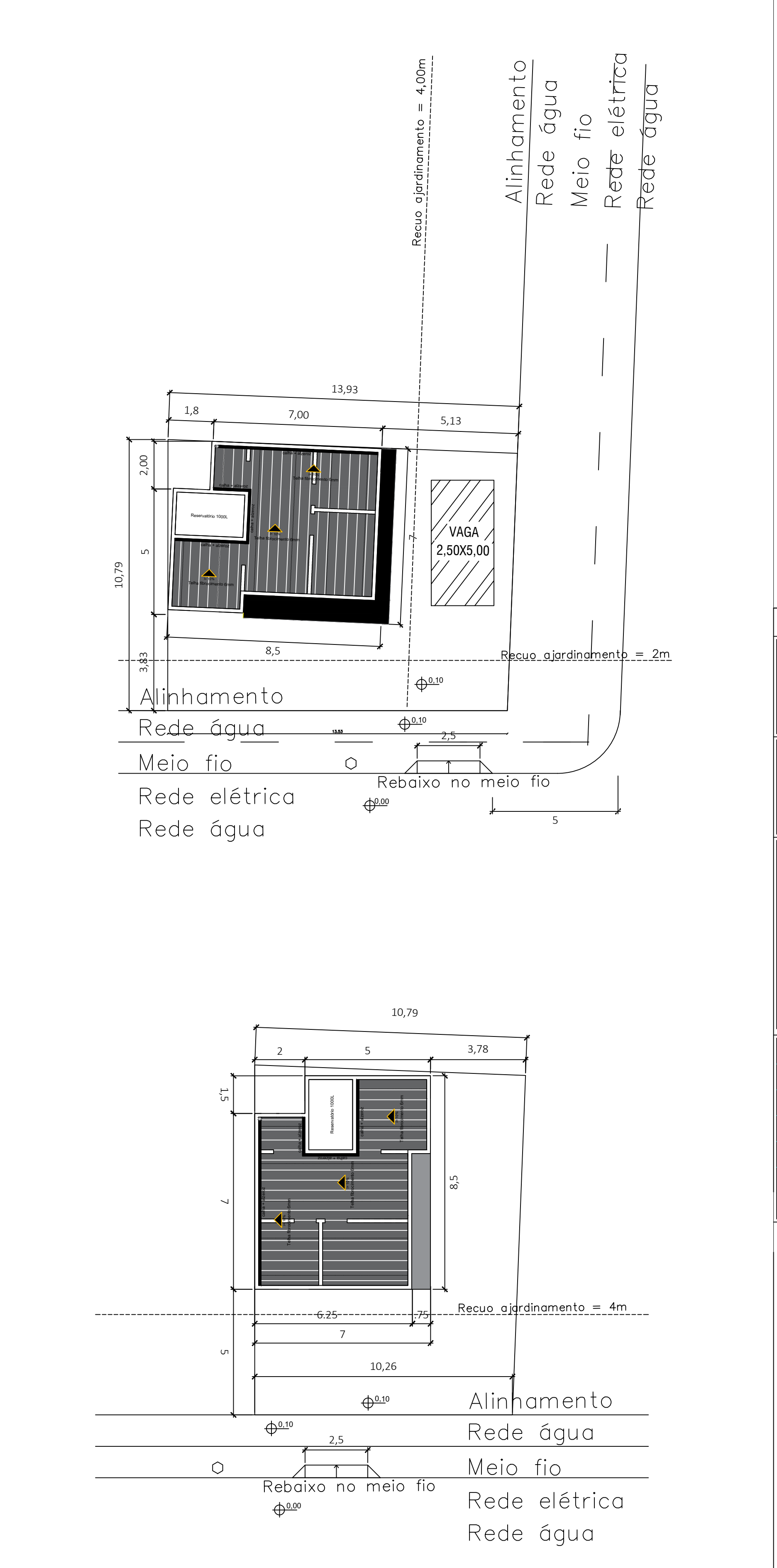
PLANTA DE SITUAÇÃO DO(S) LOTE(S) – MODELO 2 – 56,50m² Escala 1 : 125
